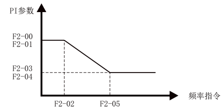
图5-18 PI参数示意图
