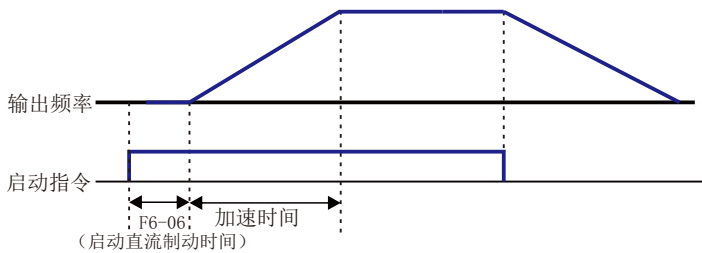
图 5-10 带直流制动的启动时序图
