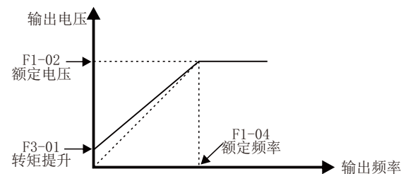
图 5-13 通用恒转矩直线 V/F 曲线
