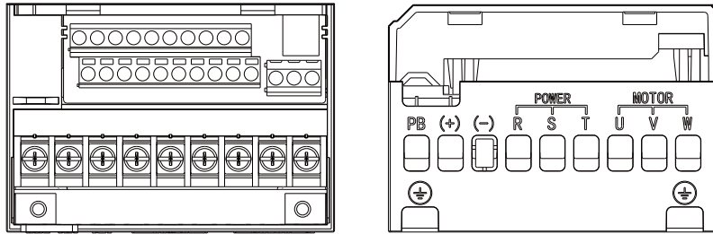
端子分布图 1
