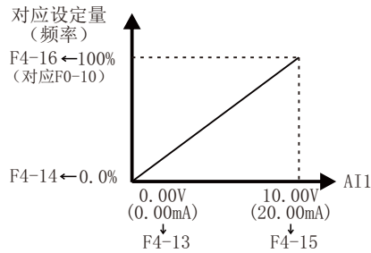
图5-1 AI 曲线 1 设定
