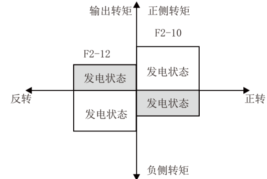
图 5-19 速度控制转矩上限示意图
