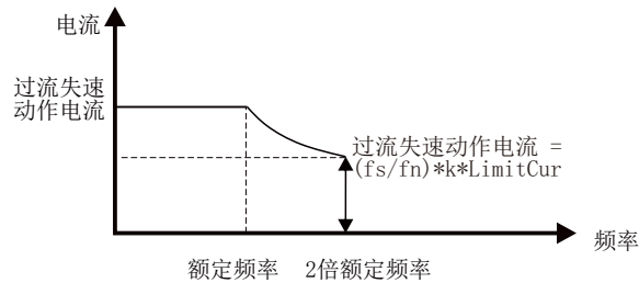
图5-17倍速过流失速动作示意图
