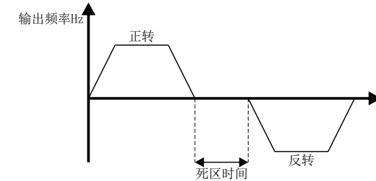
图 5-26 正反转死区时间示意图
