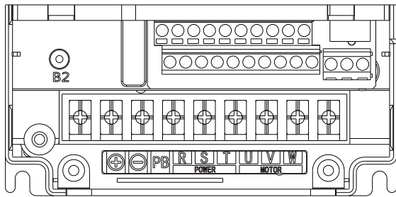
端子分布图 2
