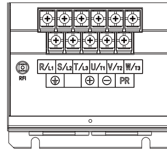
端子分布图 4
