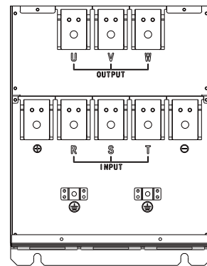
端子分布图 6
