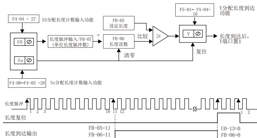
图 5-21 计数功能示意图
