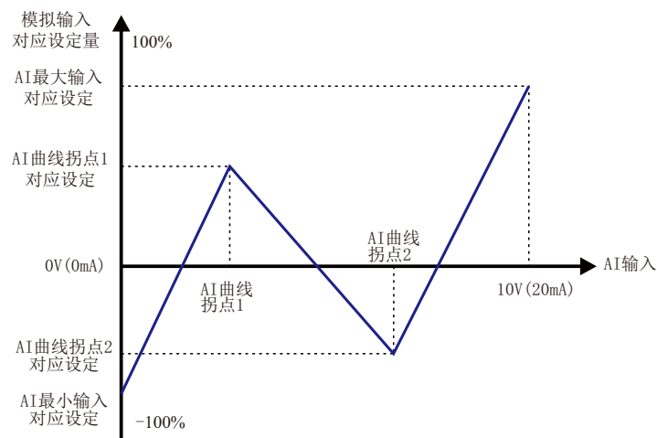
图5-3 曲线 4 和曲线 5 示意图
