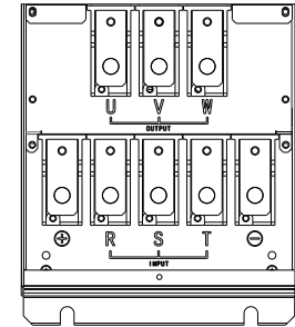
端子分布图 5
