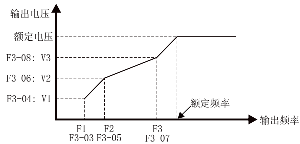
图5-14 自定义多点 V/F 曲线
