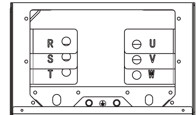
端子分布图 7
