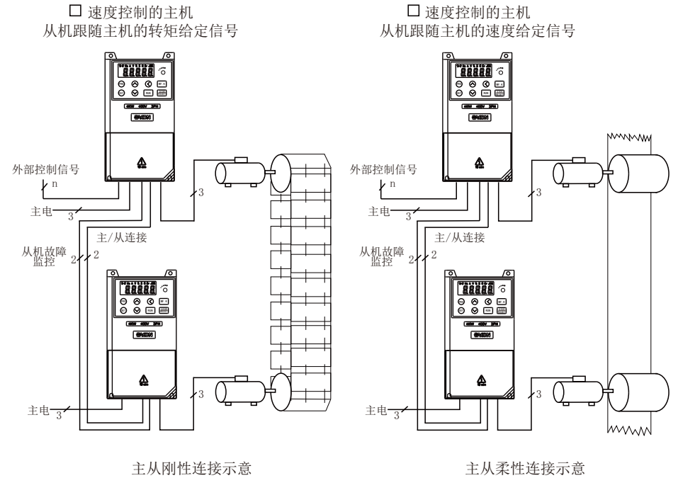
图 5-22 主从连接示意图
