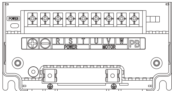
端子分布图 3
