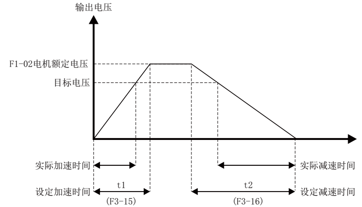
图5-15 V/F分离示意图
