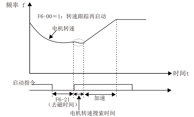
图 5-11 转速跟踪再启动方式
